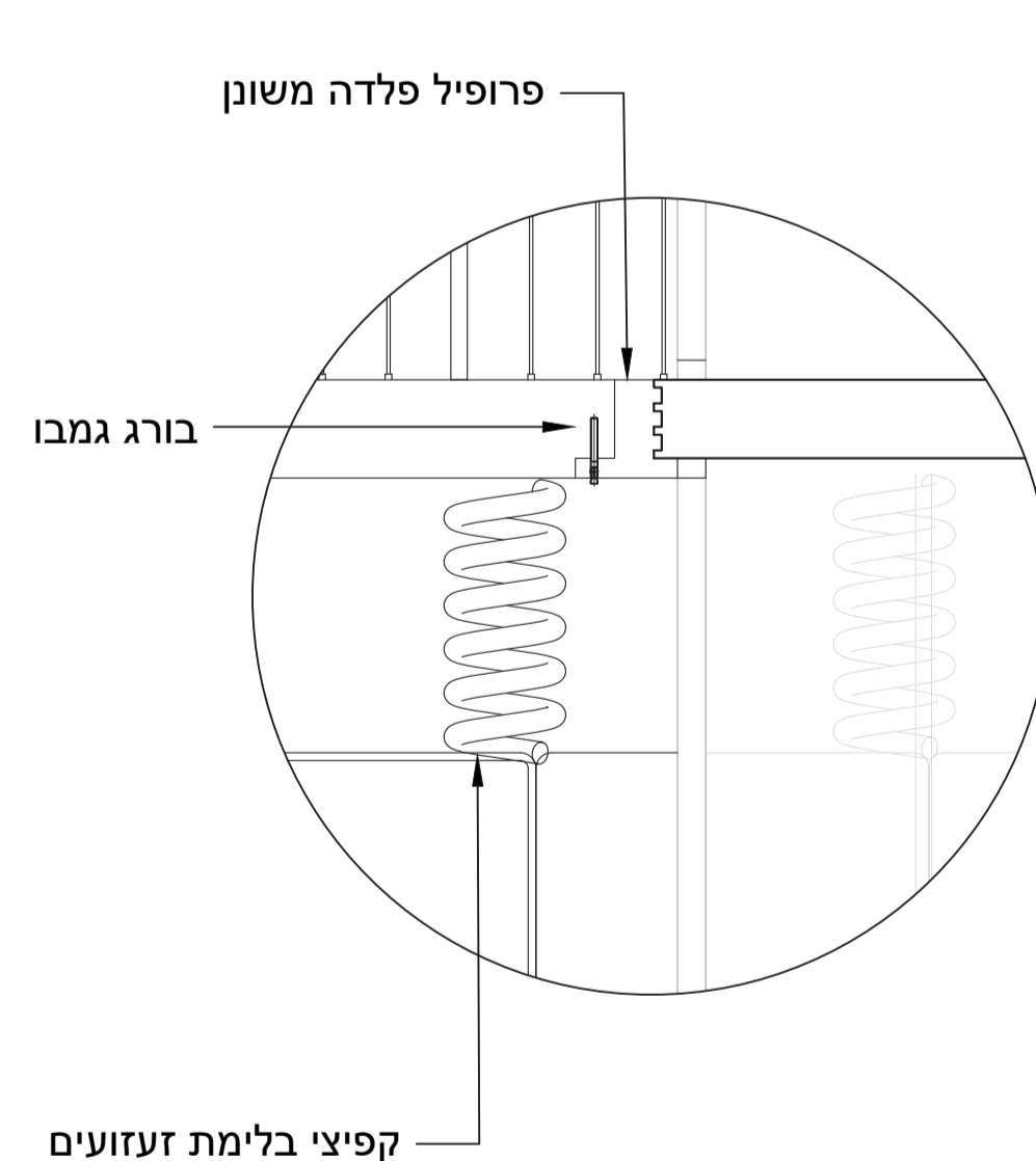
פרט חיבור טבעת קונסטרוקציה
