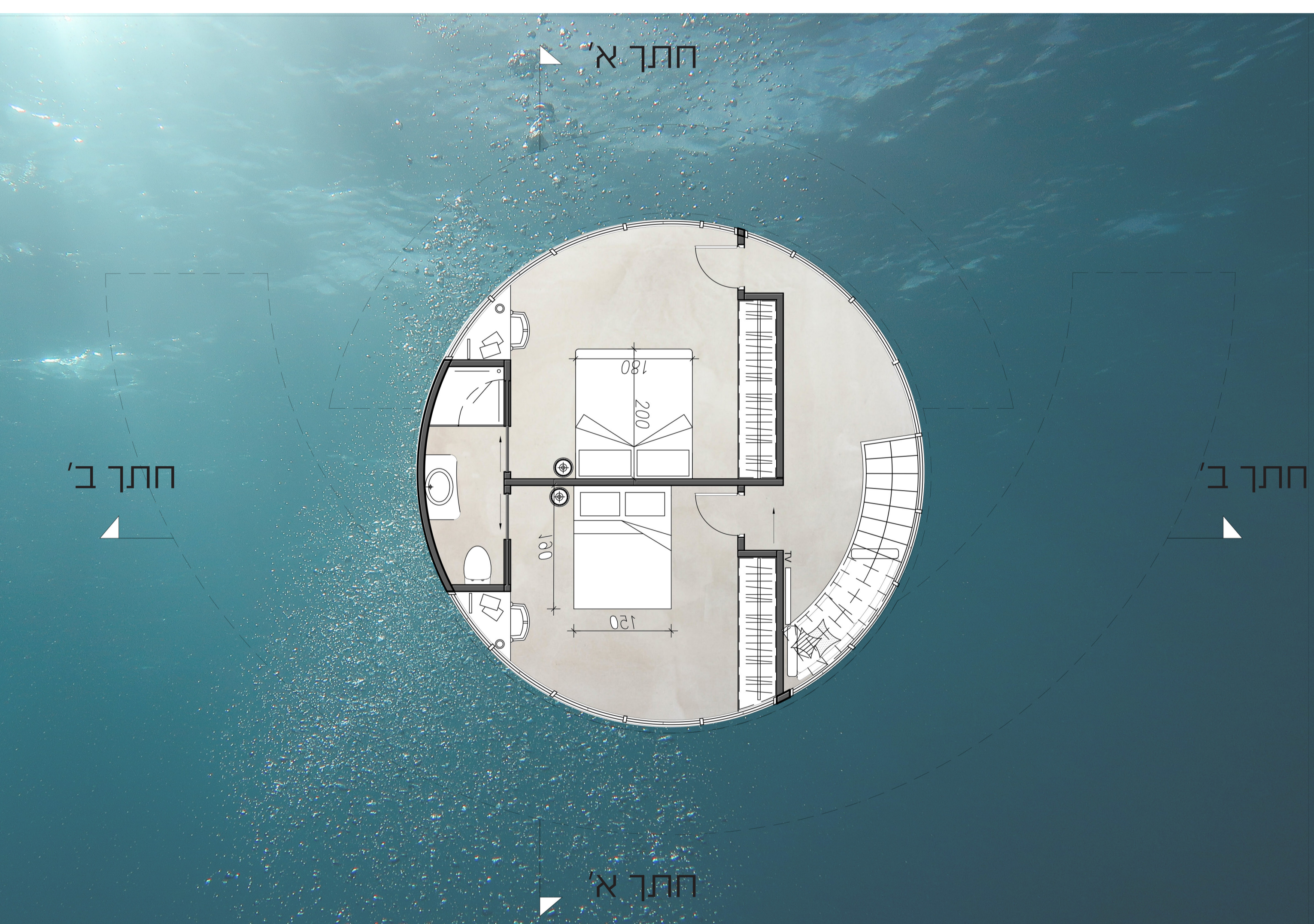
תכנית מפלס -1 יח' דיור 3 חדרים 48 מ"ר
