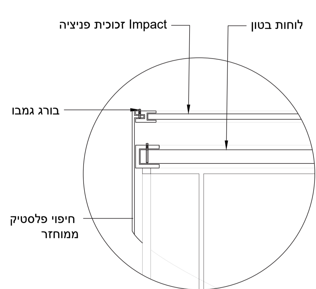
פרט חיבור חיפוי גג
