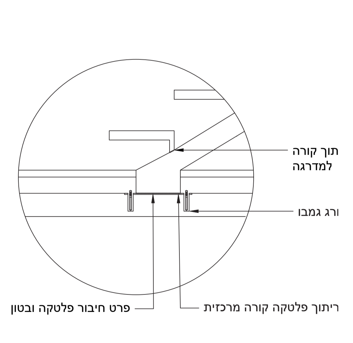
פרט חיבור רצפה
