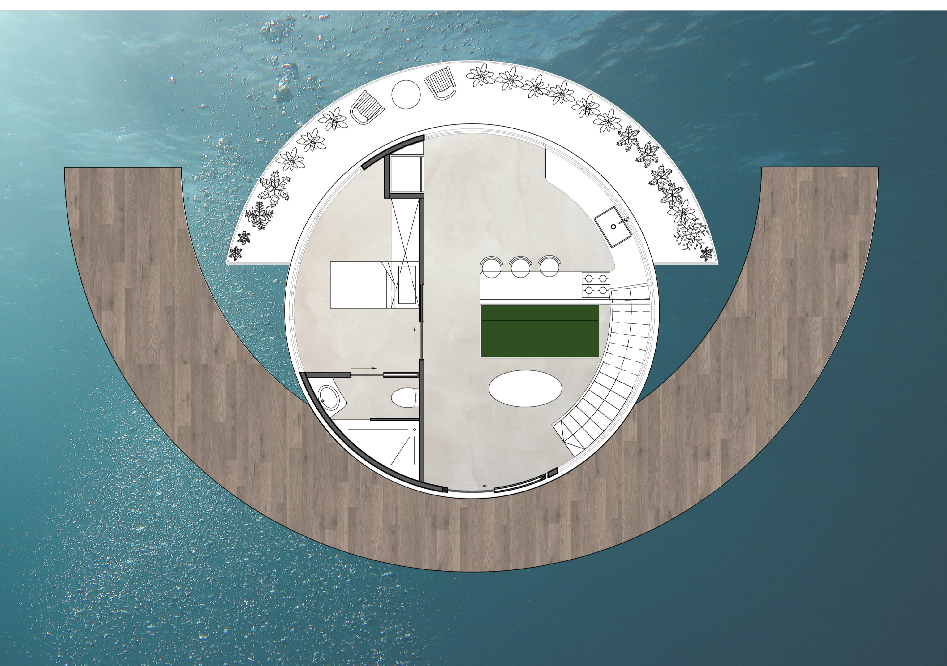
תכנית מפלס 0 יח' דיור 4 חדרים 48 מ"ר
