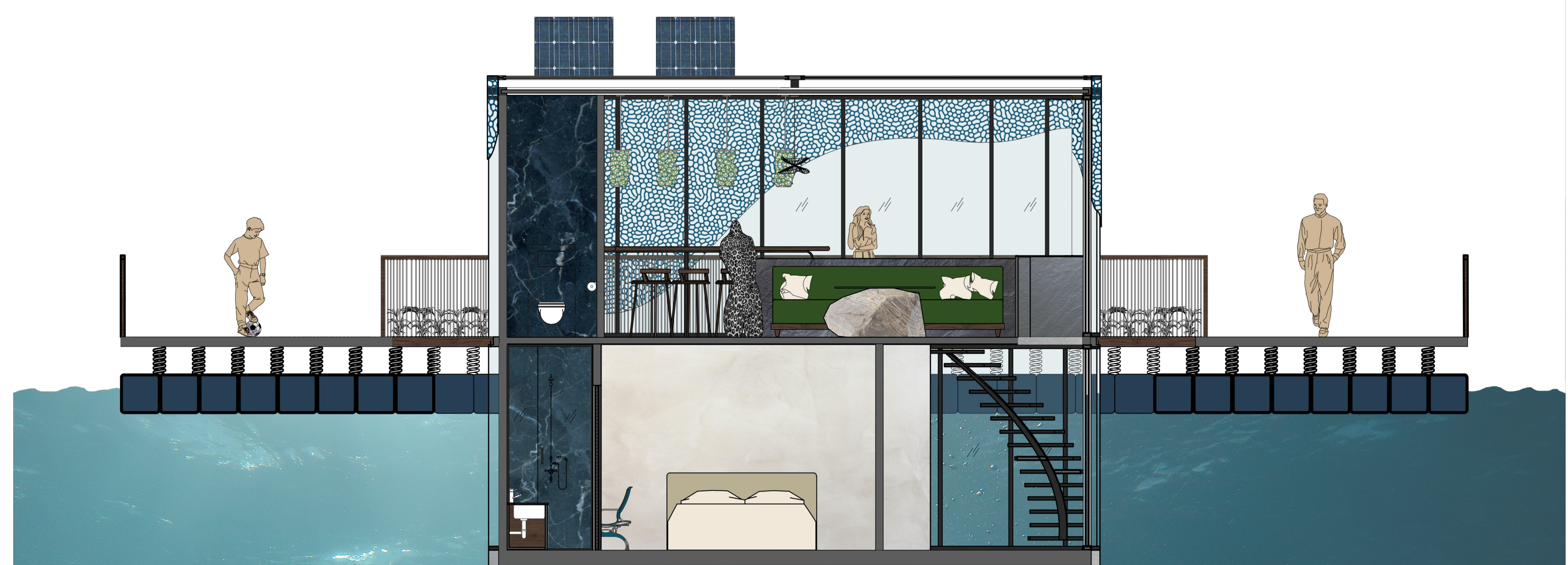
חתך - ב'
