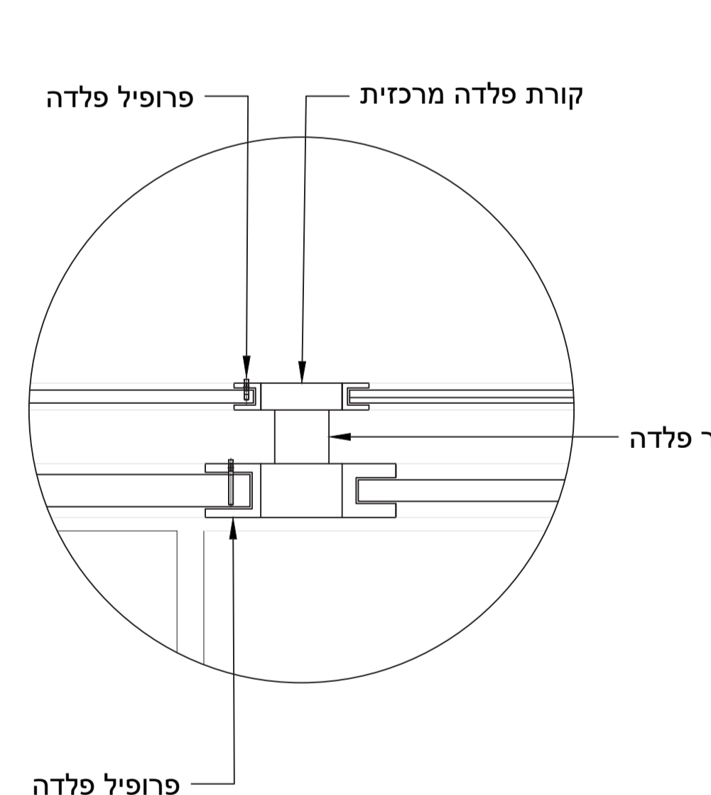
פרט חיבור גגות
