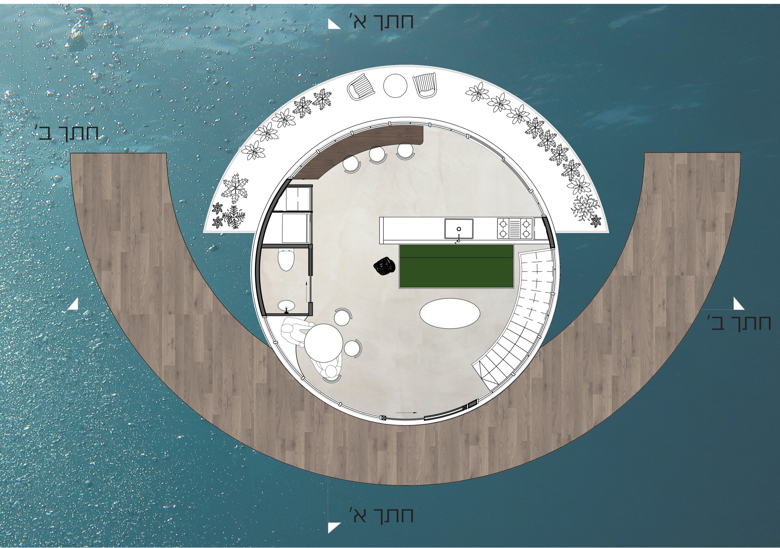
תכנית מפלס 0 יח' דיור 3 חדרים 48 מ"ר
